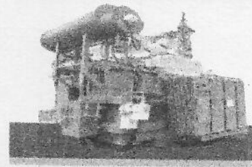
หม้อแปลงไฟฟ้ากำลังแบบปรับเปลี่ยนแรงดัน โดยอัตโนมัติ ระบบ 22 kV (Automatic Voltage Regulator (AVR) for 22 kV) - ขนาด 16 MVA (400 A) 11,277,000 บาท/เครื่อง
